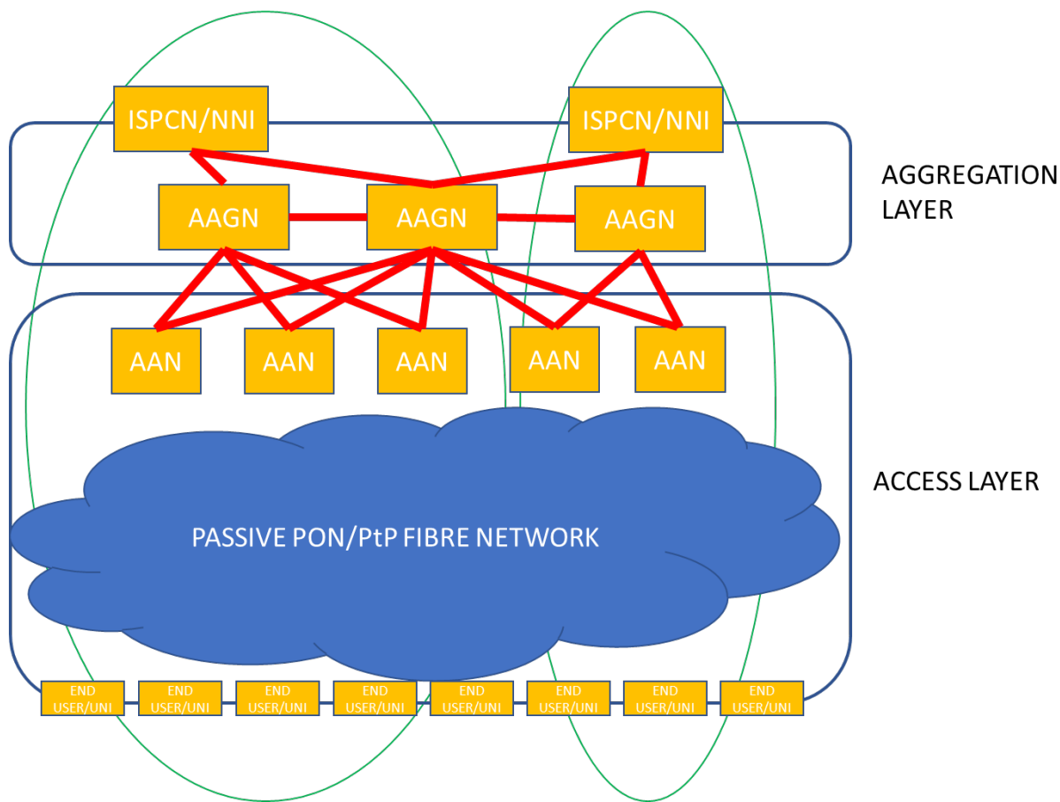
Slika 1: Topologija dostopnega kablanskega omrežja
